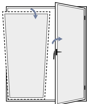
Porte-fenêtre 2 vantaux oscillo-battant
